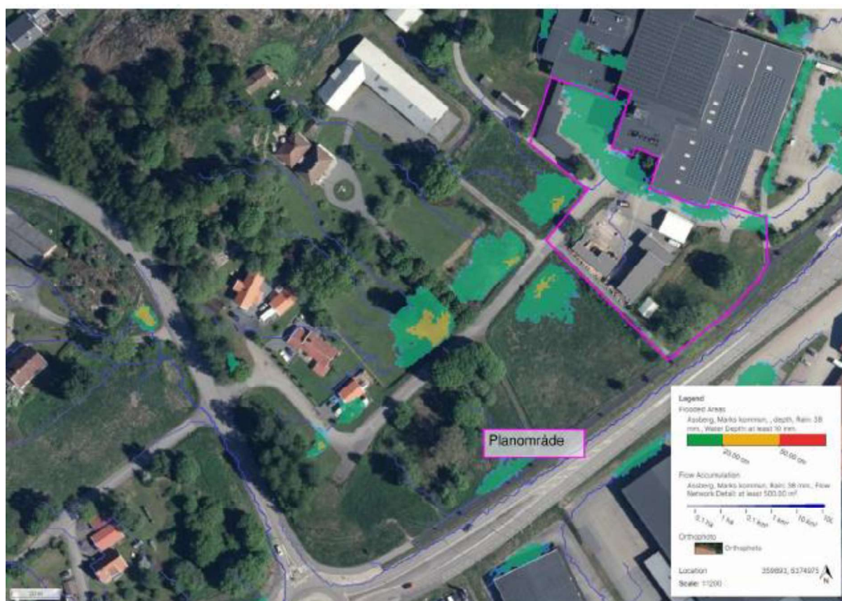
Figur 23. En analys av befintliga förhållanden vid skyfall vid ett 100 års regn, 10 minuters varaktighet, klimatkfaktor 1,3 och ett vattendjup på upp till 20 cm (grönt område).
