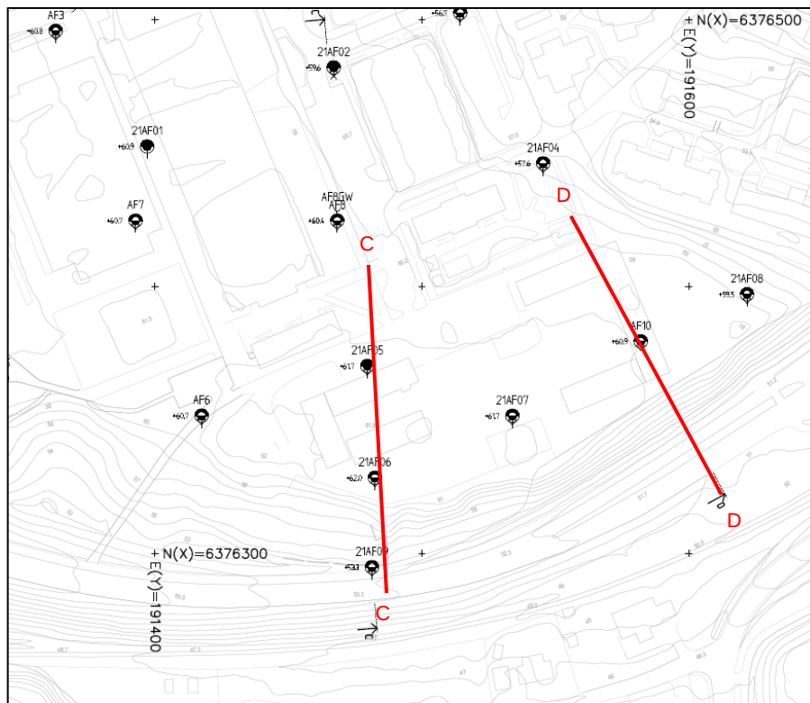
Figur 6.1. Beräkningssektionernas läge för stabilitetsutvärdering.
