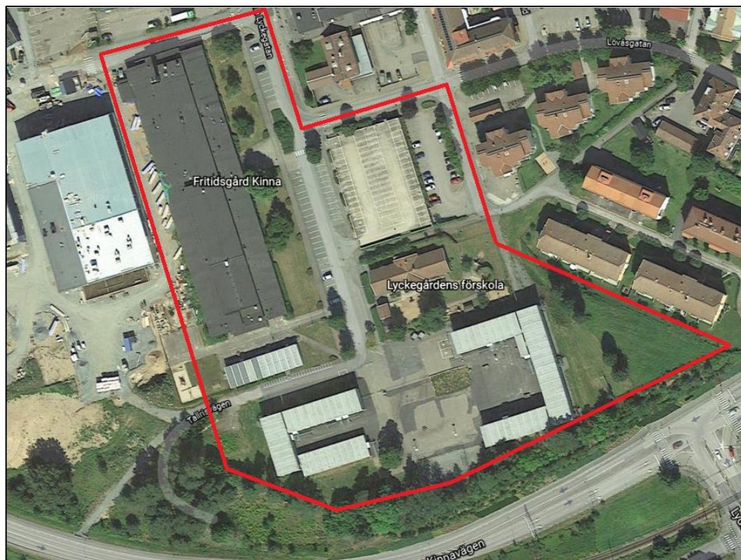
Figur 5.1. Satellitkarta över undersökningsområdet i Kinna, Marks kommun. Områdesgränsen är markerad med rött. (Hämtat från Google Earth 2021-09-09).
