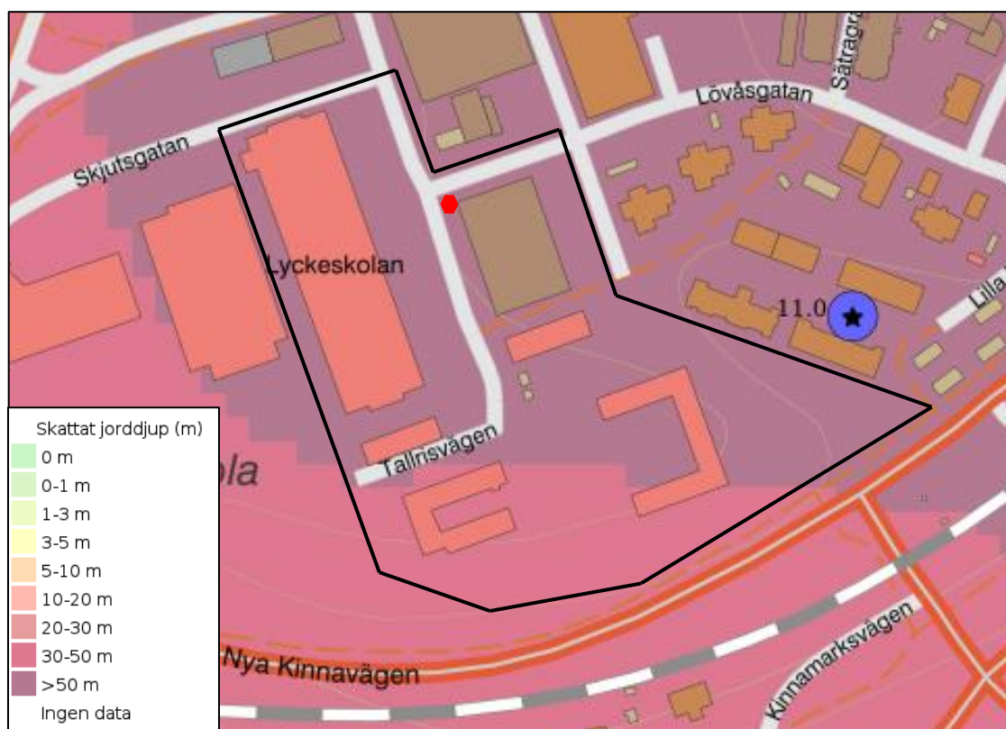
Figur 5.2. Urklipp från SGU:s jorrdjupskarta med undersökningsområde markerat i svart (Hämtat från SGU:s kartvisare 2021-09-21).
