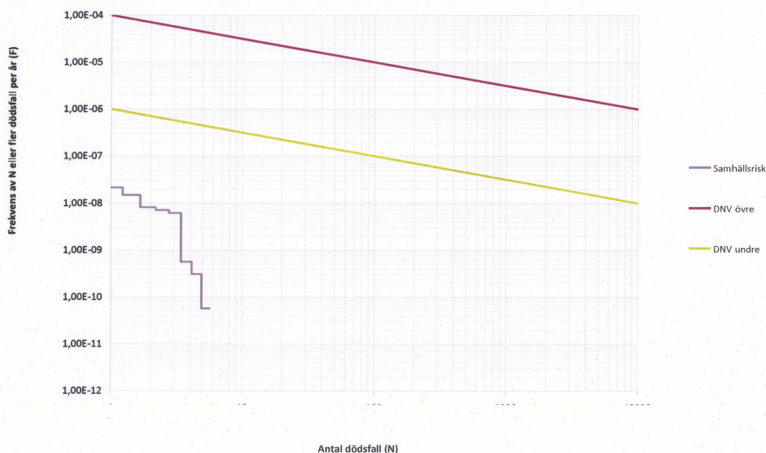
Figur 13 Samhällsrisk i form av FN-kurva för godsflöden för 2013.
