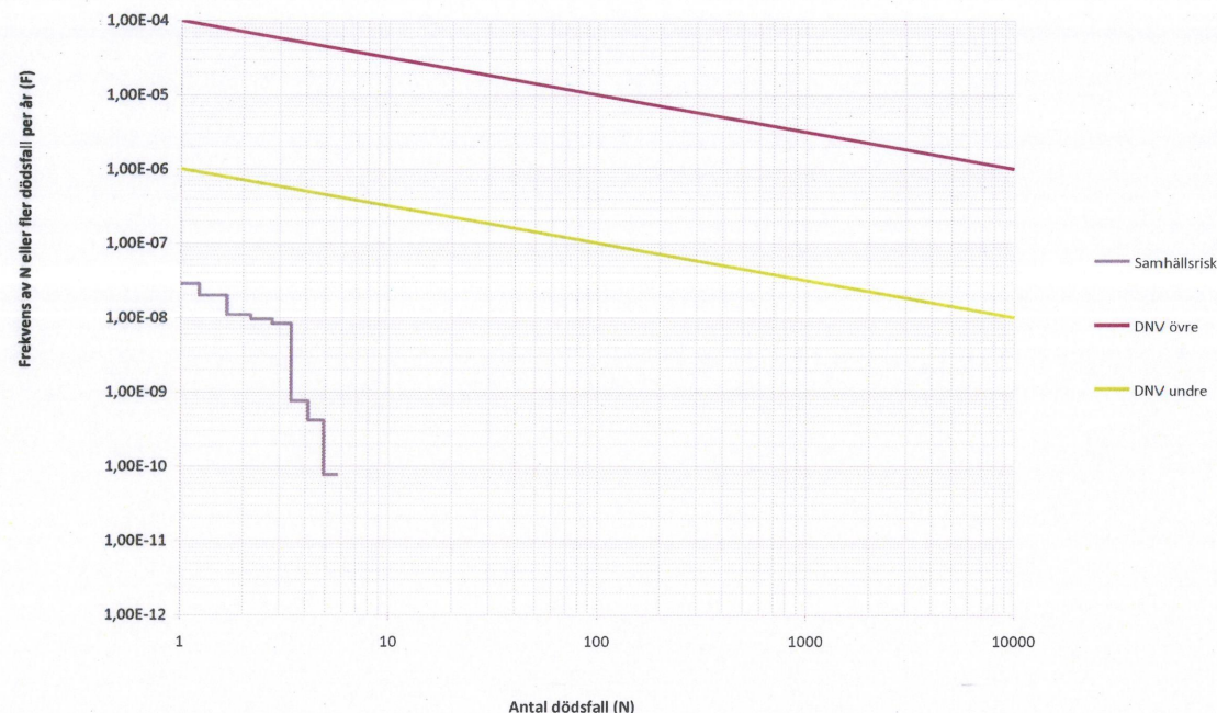
Figur 14 Samhällsrisk i form av FN-kurva för godsflöden uppskattade för 2034.
