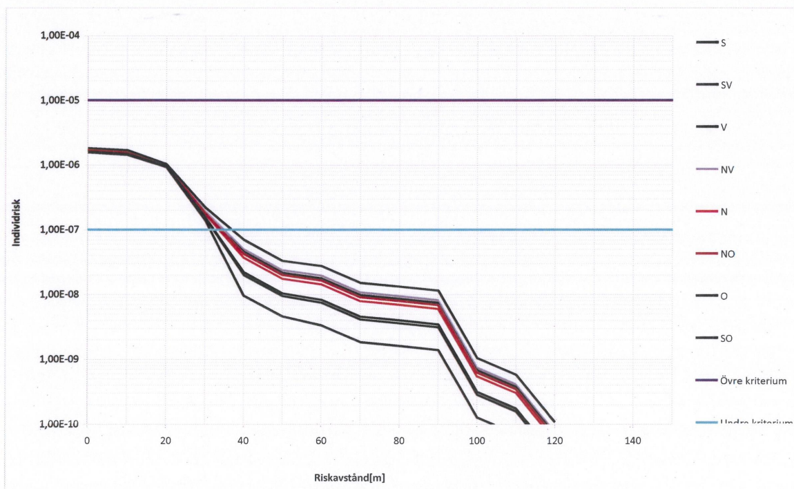
Figur 12 Individerisk för prognostiserade godsflöden år 2034.
