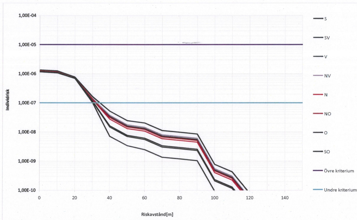
Figur 11 Individerisk för godsflöden enligt dagens nivåer
