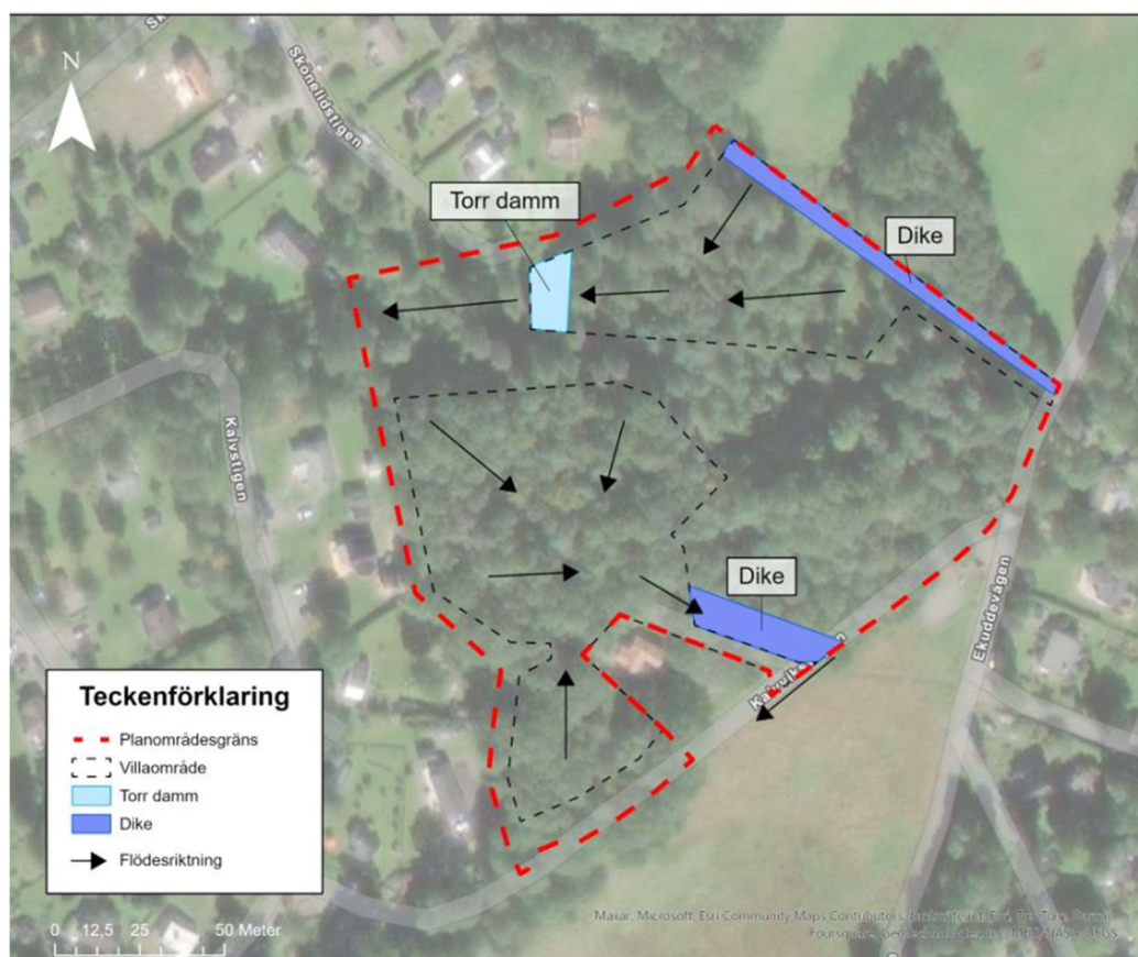
Figur 11: Föreslagen placering av dagvattenanläggningar enligt genomförd dagvattenutredning, Sweco.
