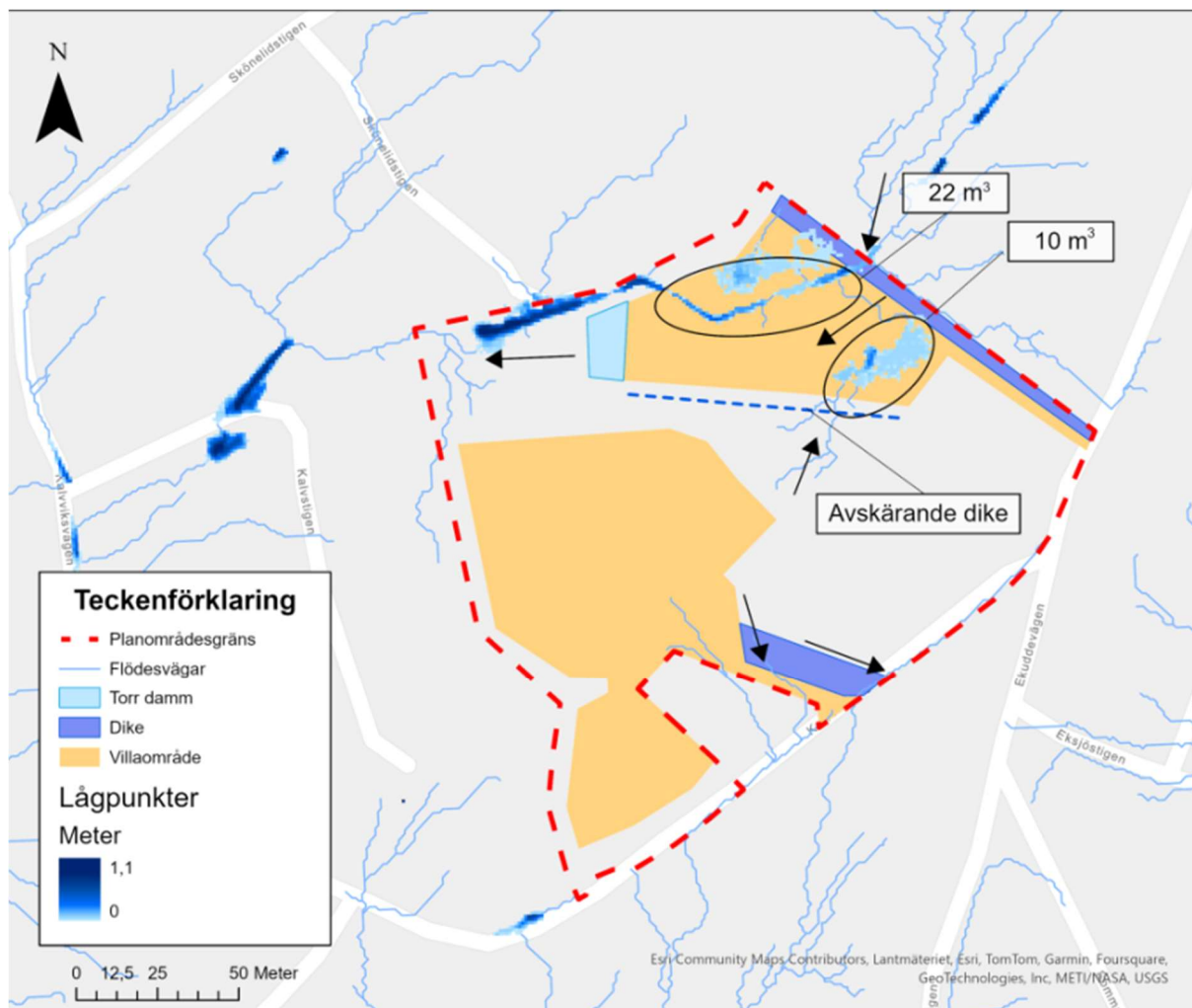
Figur 12: Avskärande diken för att skydda bebyggelse inom planområdet från vatten vid skyfall, Sweco.
