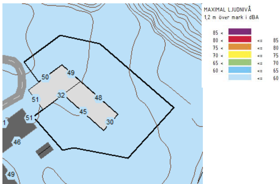
Figur 12. Maximal ljudutbredning 1,5m över mark från industri. Förskolegård dagtid vardagar kl.06 – 18.
