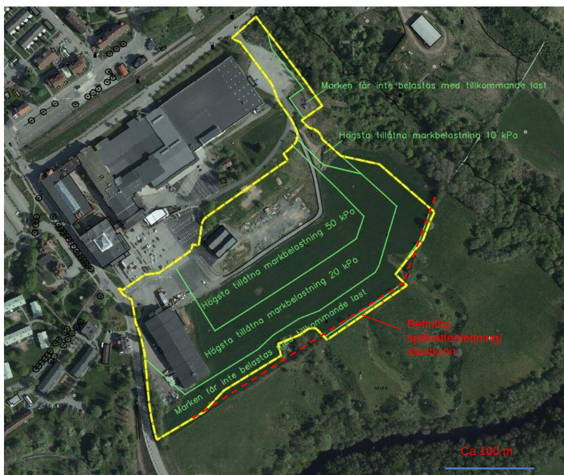
Figur 26 – Föreslagna belastningsrestriktioner med hänsyn till geotekniska förhållanden. Ortofoto källa: www.lantmateriet.se .
